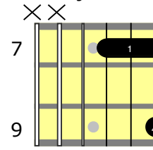
Dmaj7
