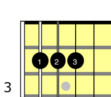
Esus4
